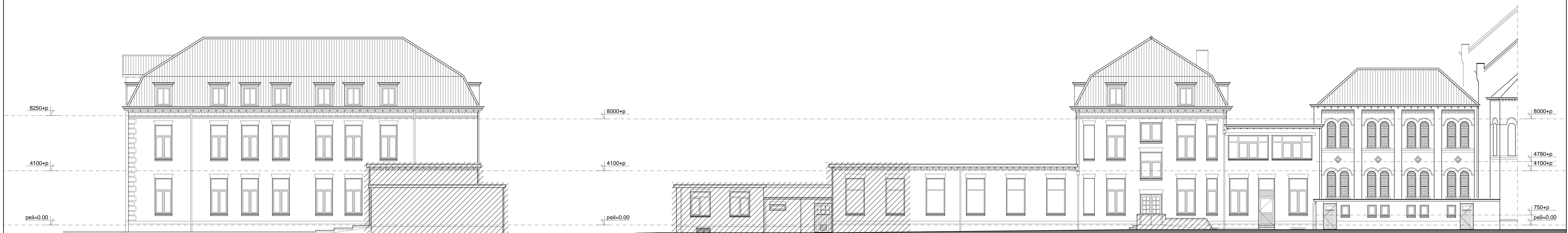
linker zijgevel
