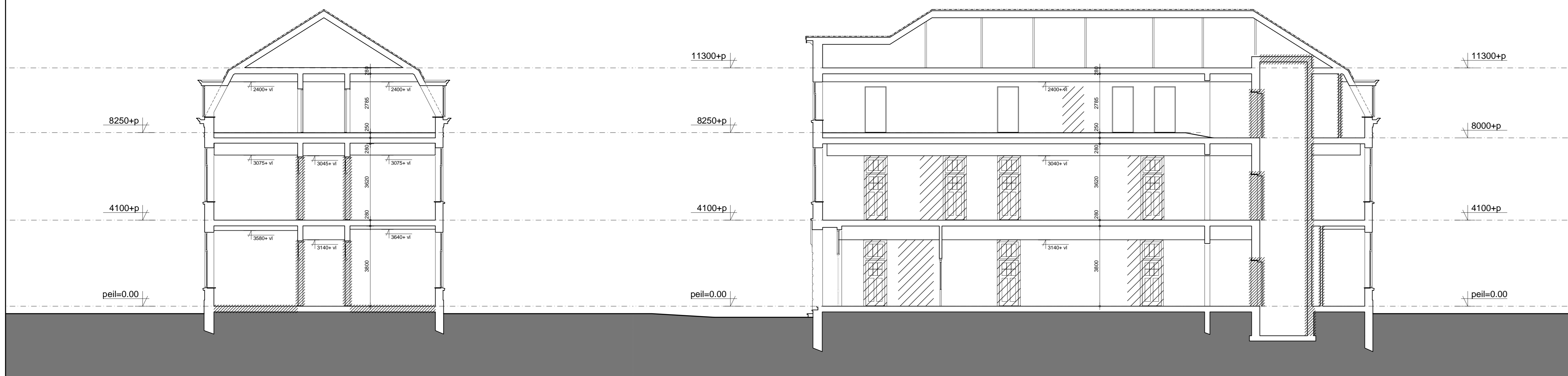
doorsnede b-b
